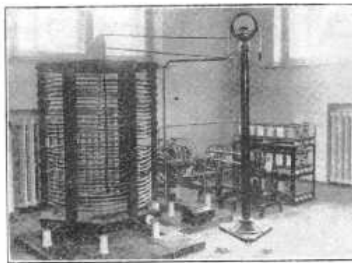
De antennespoel
