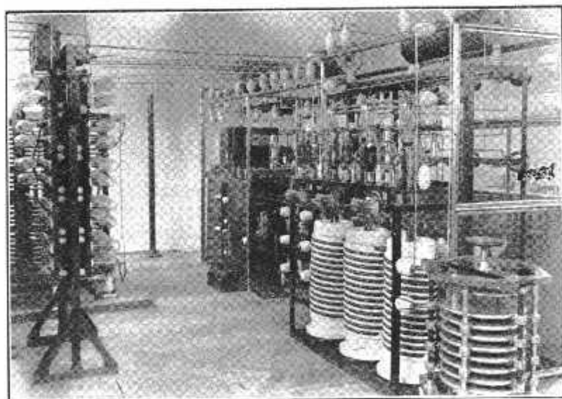
De opstelling der watergekoelde zendlampen
