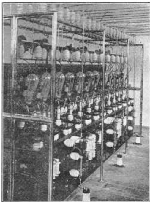
De gelijkrichter-installatie
